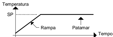
Figura 4 - Função Rampa ao Patamar
