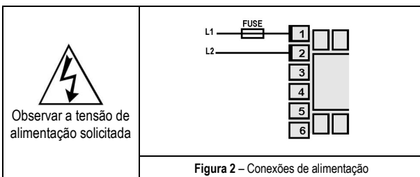
Figura 2 – Conexões de alimentação
