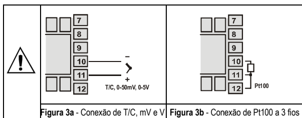
Figura 3a - Conexão de T/C, mV e V
