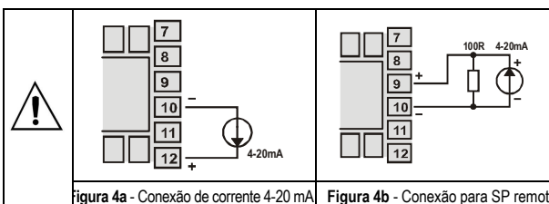
Figura 4a - Conexão de corrente 4-20 mA
