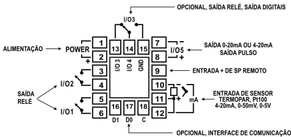
Figura 1 - Conexões do painel traseiro
