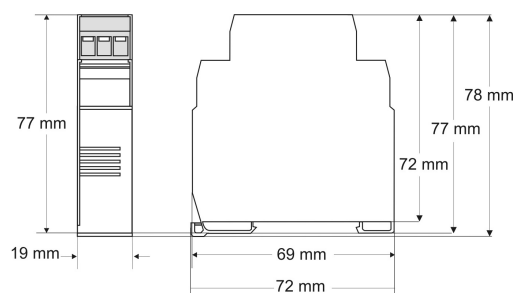
Figura 1 – Dimensões
