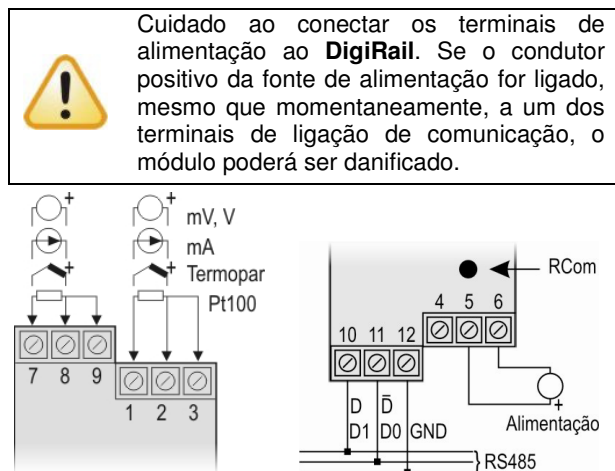
Figura 2 – Conexões Elétricas
