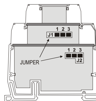
Figura 3 – Jumper para entrada 0-5 Vcc e 0-10 Vcc
