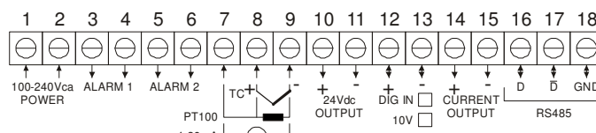
Figura 3 - Conexões do painel traseiro
