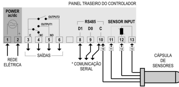
Figura 02 - Conexões mostradas na etiqueta do controlador - Reles não isolados - Modelo Padrão
