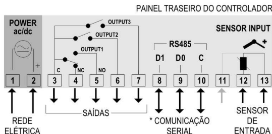
Figura 01 – Conexões mostradas na etiqueta do controlador
